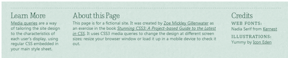
Рис. 7.13. Несмотря на то что в коде HTML div-блок learn-more находится между div-блоками about и credits , значение его свойства box-ordinal-group заставляет браузер выводить этот блок у левого края страницы
