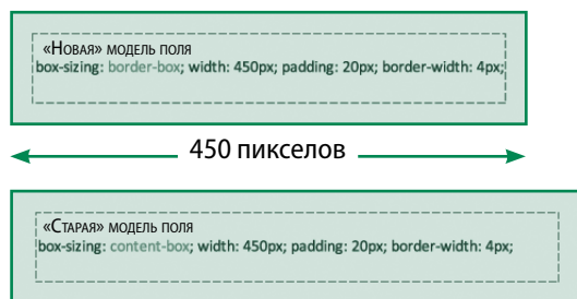
Рис. 7.28. Различие между content-box и border-box заключается в том, какой размер определяет значение свойства width : ширину области содержимого или ширину всего поля от рамки до рамки
