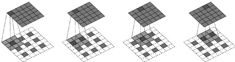
Рис. 15.1. Транспонированная свертка (изображение любезно предоставлено Винсентом Дюмулином и Франческо Визином)
