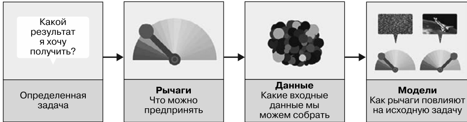
Рис. 2.2. Трансмиссионный подход
