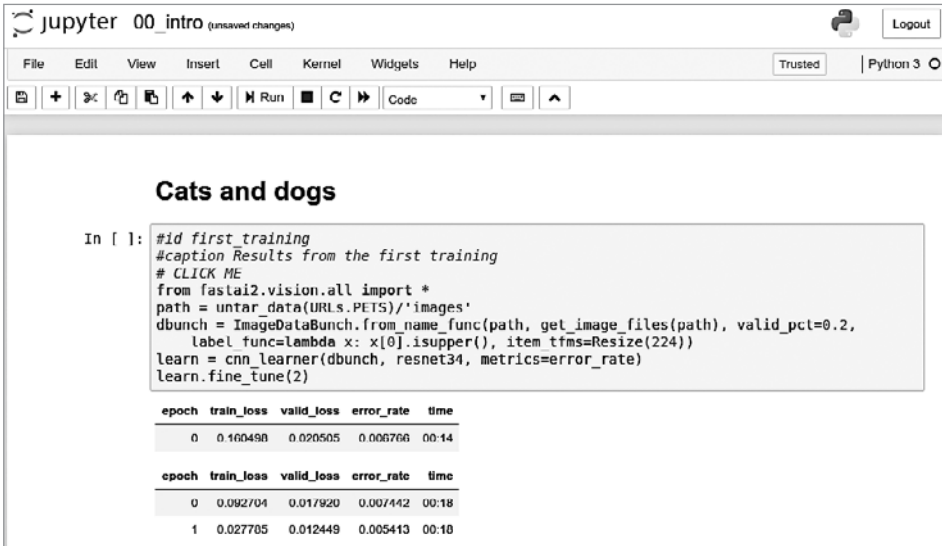
Рис. 1.3. Блокнот Jupyter
