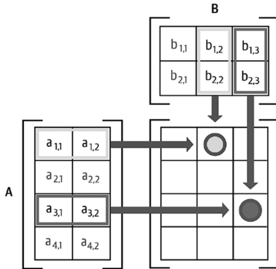
Рис. 4.6. Матричное умножение
