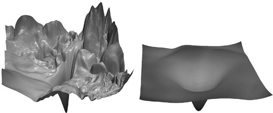
Рис. 14.3. Влияние ResNet на ландшафт потерь (изображение любезно предоставлено Хао Ли и др.)
