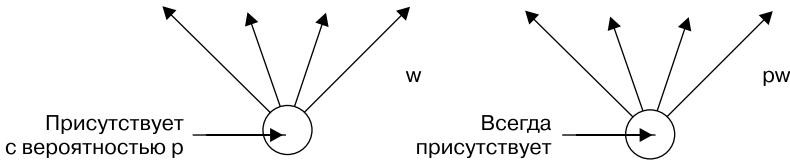
Рис. 12.11. Почему мы масштабируем активации при применении дропаута (изображение любезно предоставлено Нитишем Шриваставой (Nitish Srivastava) и др.). Слева: блок во время обучения, который присутствует с вероятностью p и связан с блоками в следующем слое с весами w . Справа: во время тестирования этот блок присутствует всегда, и веса умножаются на p . Вывод при тестировании такой же, что и ожидаемый вывод при обучении
