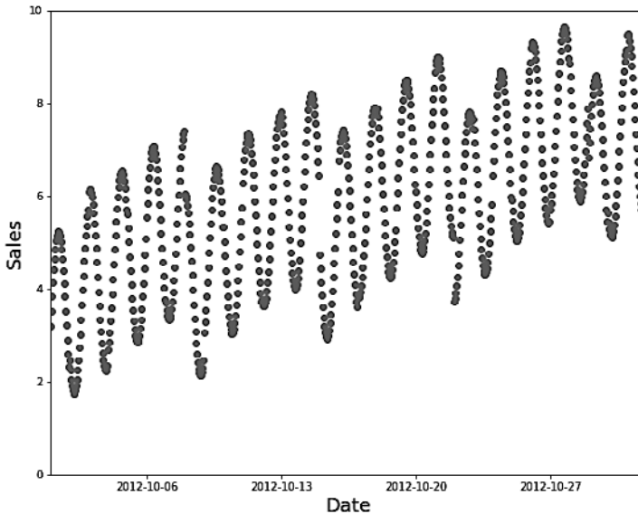
Рис. 1.19. Временной ряд
