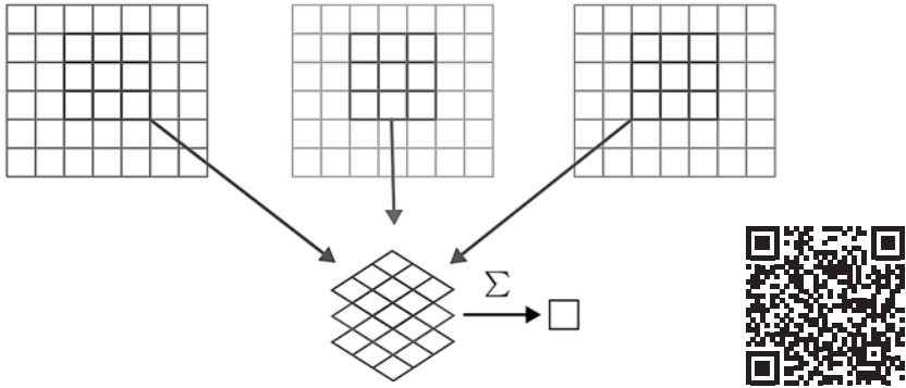
Рис. 13.13. Сложение RGB-фильтров
