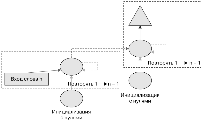
Рис. 12.6. Двуслойная RNN
