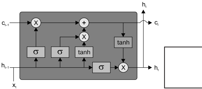
Рис. 12.9. Архитектура LSTM
