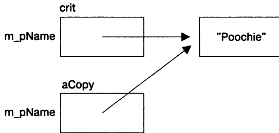
Рис. 9.8. Если бы была создана поверхностная копия объекта crit , объекты aCrit и crit имели бы члены данных, указывающие на один фрагмент памяти
