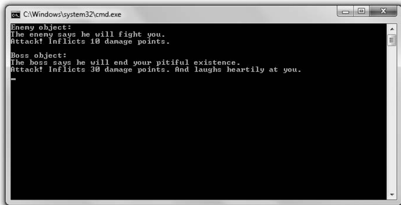
Рис. 10.3. Класс Boss наследует и переопределяет функции-члены базового класса Taunt() и Attack() , создавая тем самым новое поведение этих функций для класса Boss (опубликовано с разрешения компании Microsoft)
