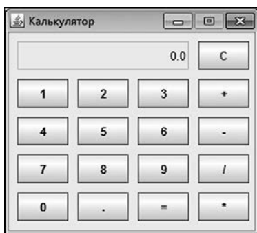
Рис. 12.12. Окно программы-калькулятора
