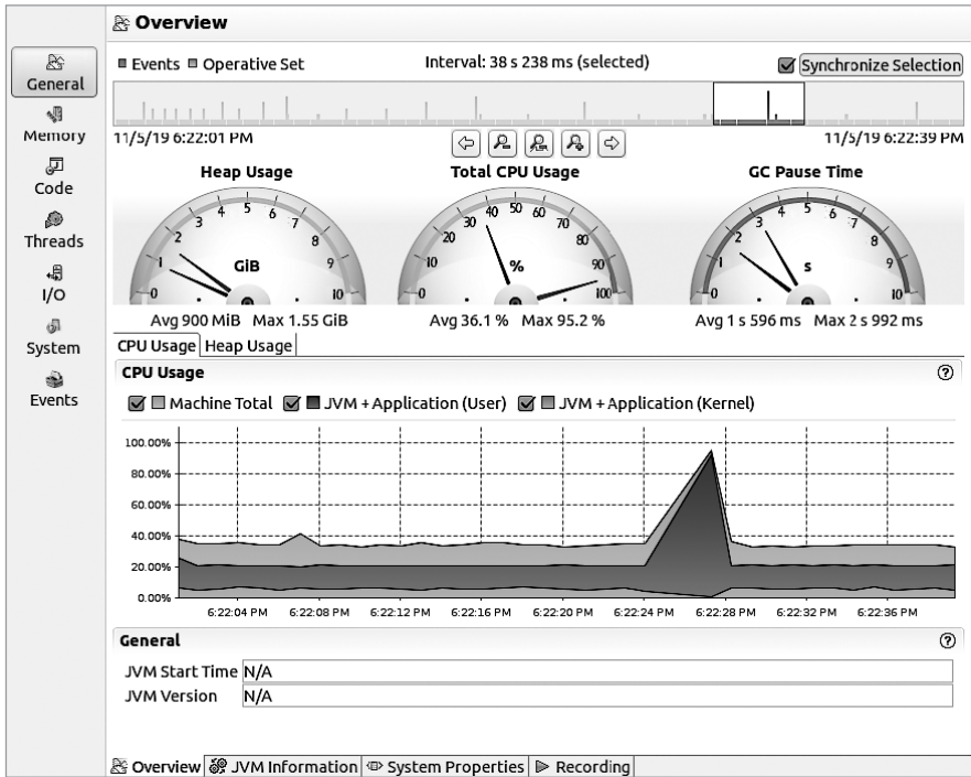
Рис. 3.10. Общая информация в JFR
