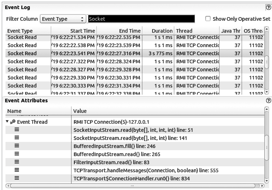
Рис. 3.14. Панель Log в JFR
