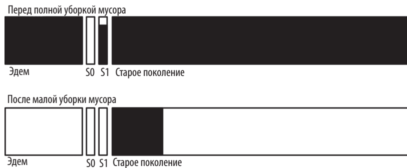
Рис. 6.2. Параллельная полная уборка мусора
