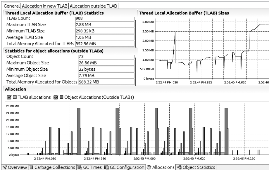
Рис. 6.10. Избыточное выделение памяти за пределами TLAB
