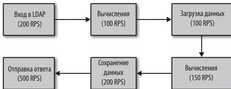
Рис. 2.1. Типичный поток выполнения программы
