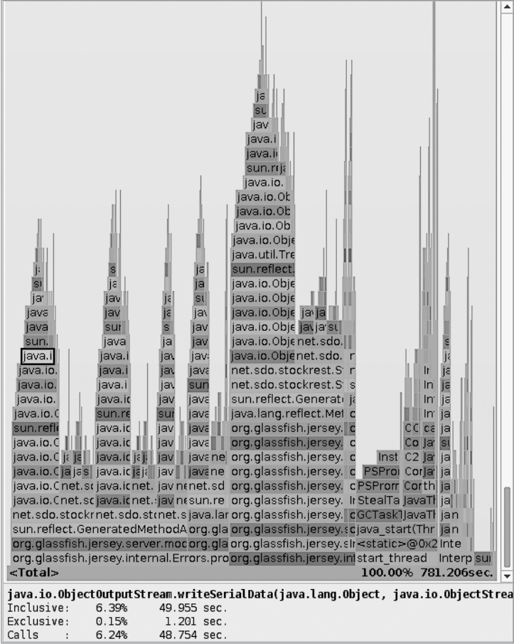
Рис. 3.8. Огненный график с включением низкоуровневого кода
