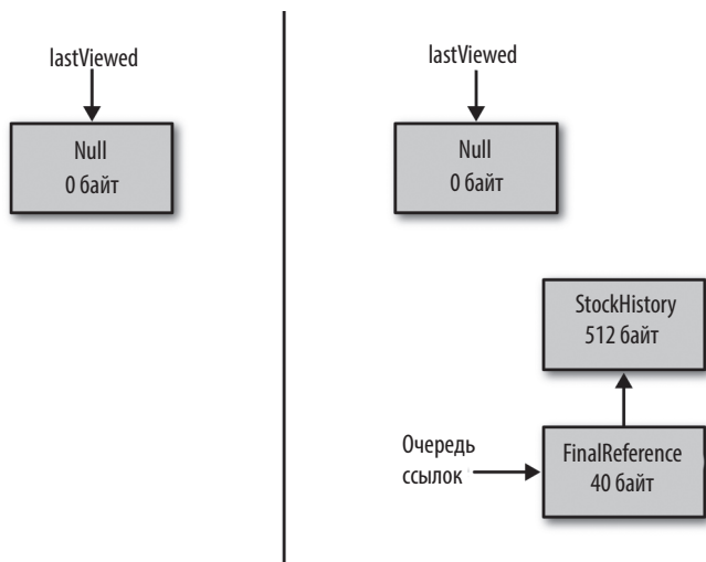
Рис. 7.9. Финальные ссылки удерживают больше памяти
