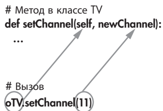
Рис. 2.5. Вызов метода
