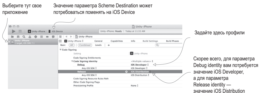
Рис. 13.4. Настройка профилей в интегрированной среде разработки Xcode
