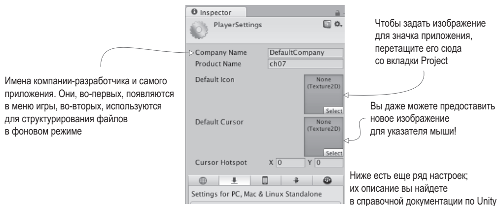
Рис. 13.2. Настройки проигрывателя на панели Inspector
