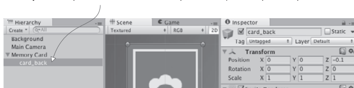
Рис. 5.6. Иерархическое связывание и местоположение спрайта с рубашкой карты
