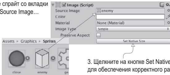
Рис. 7.6. Назначение двумерных спрайтов свойству Image элементов интерфейса
