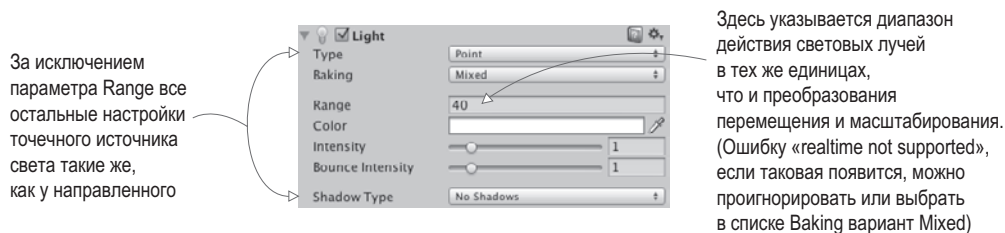
Рис. 2.9. Настройки точечного источника света на панели Inspector
