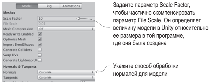
Рис. 8.4. Параметры импорта для модели персонажа
