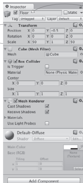
Рис. 2.6. Панель Inspector для пола
