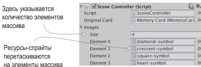
Рис. 5.8. Заполнение массива спрайтов
