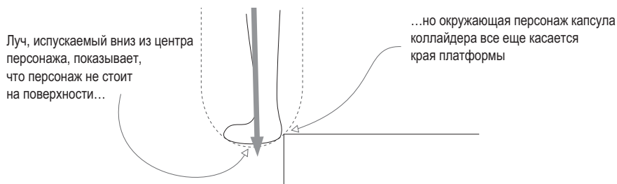
Рис. 8.10. Схема бросания лучей вниз при сходе с края платформы
