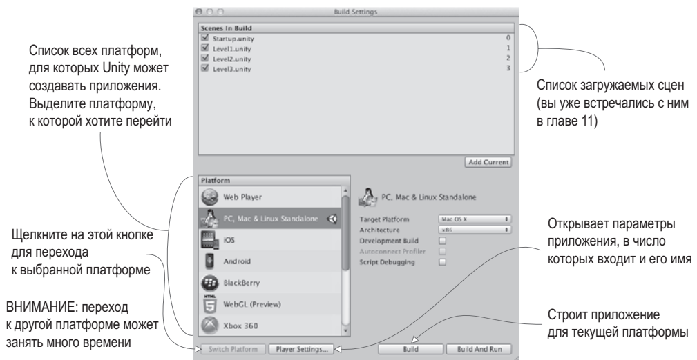
Рис. 13.1. Окно Build Settings
