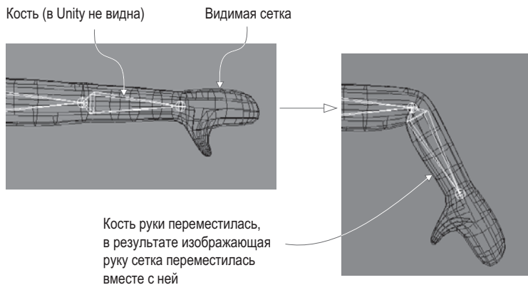
Рис. 8.12. Скелетная анимация антропоморфного персонажа
