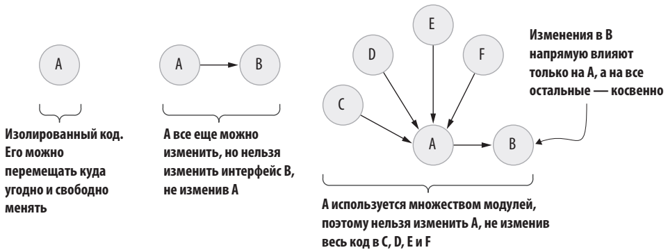
Рис. 3.2. Пригодность к изменениям обратно пропорциональна количеству зависимостей
