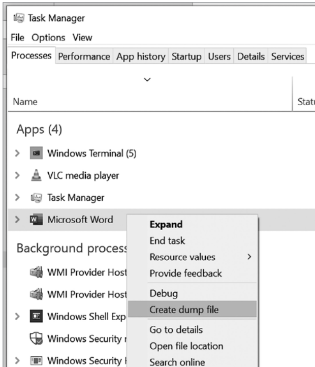
Рис. 9.4. Создание аварийного дампа работающего приложения вручную
