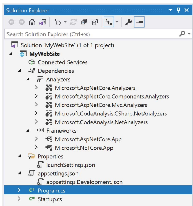
Рис. 13.2. Окно Solution Explorer
