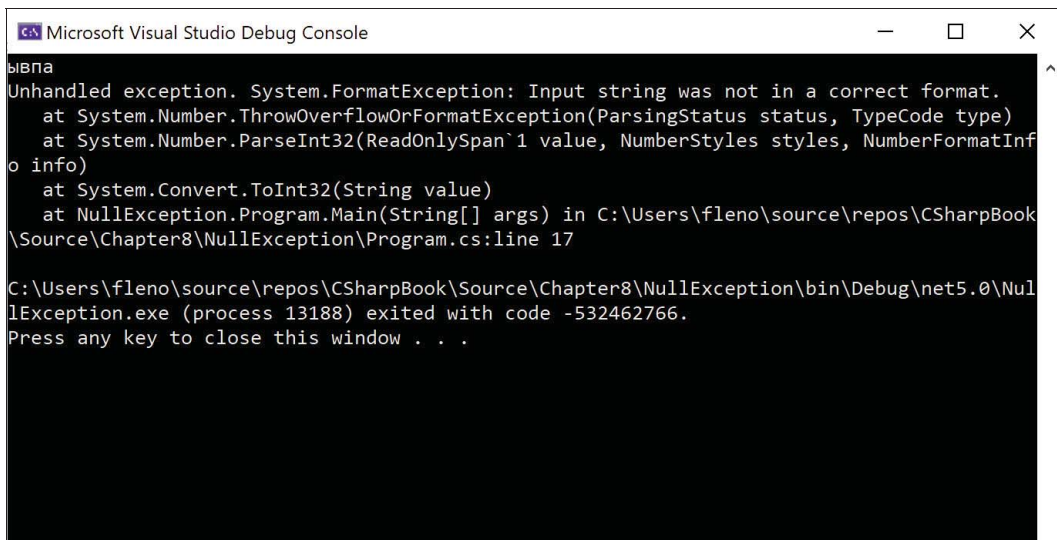
Рис. 8.1. Реакция на исключительную ситуацию при выполнении консольного приложения
