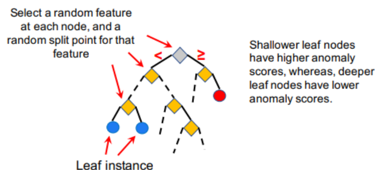
Рис. 4.10. Алгоритм деревьев изоляции (источник [Das])
