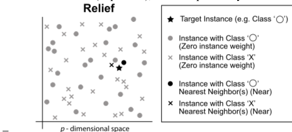
Рис. 5.2. Алгоритм Relief: выбор ближайших соседей по попаданию и промаху перед подсчетом очков
