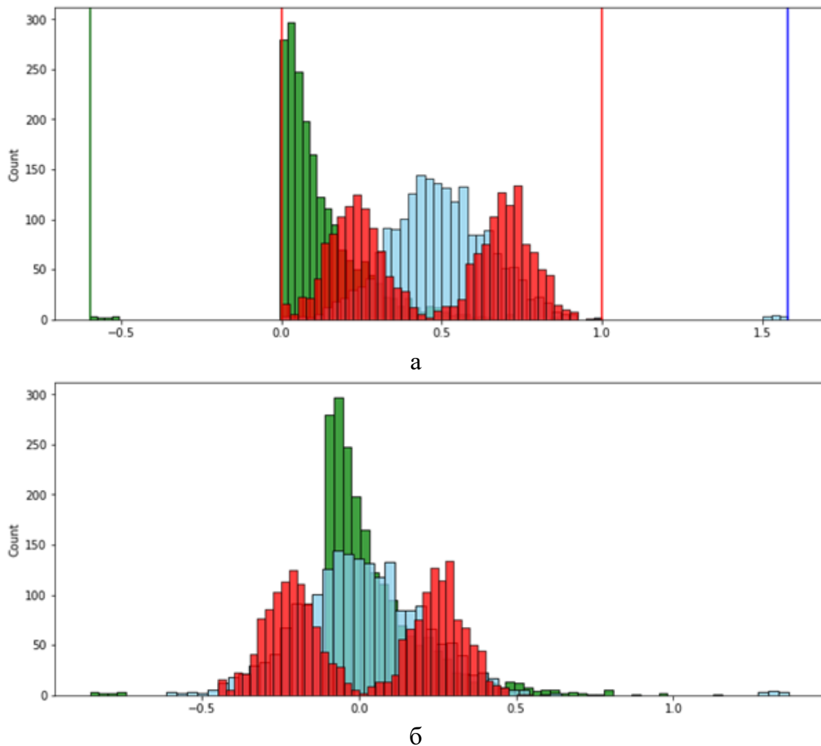
Рис. 5.4. Нормализация данных методом скорректированного интервала: а – исходные распределения, б – скорректированные распределения (источник [ https://habr.com/ru/articles/527334/ ])
