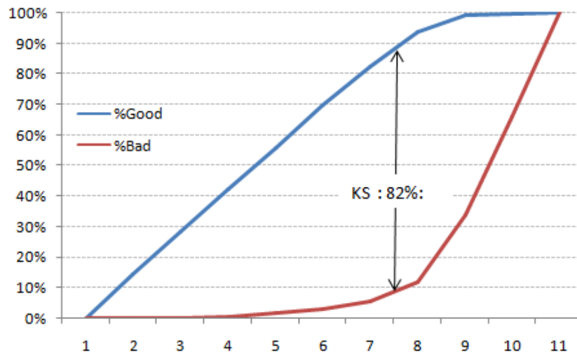
Рис. 6.4. Диаграмма Колмогорова-Смирнова
