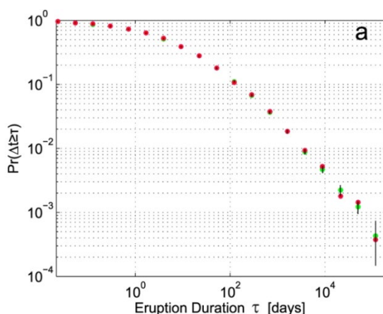
Рис. 3.27. Распределение длительности извержений вулканов
