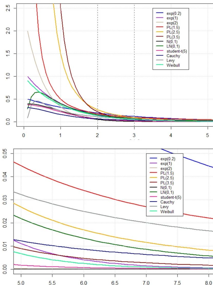
Рис. 3.25. Соотношение тяжелохвостых и легкохвостых распределений вблизи нуля (а) и на хвосте распределений (б). Обозначения: Exponential distribution (exp), Power-law distribution (PL), Normal distribution (N), Log-Normal distribution (LN), Student-t distribution, Cauchy distribution, Levy distribution, Weibull distribution (источник [https://towardsdatascience.com/journey-to-tempered-stable-distribution-part-1-fat-tailed-distribution-958d28bc20c])
