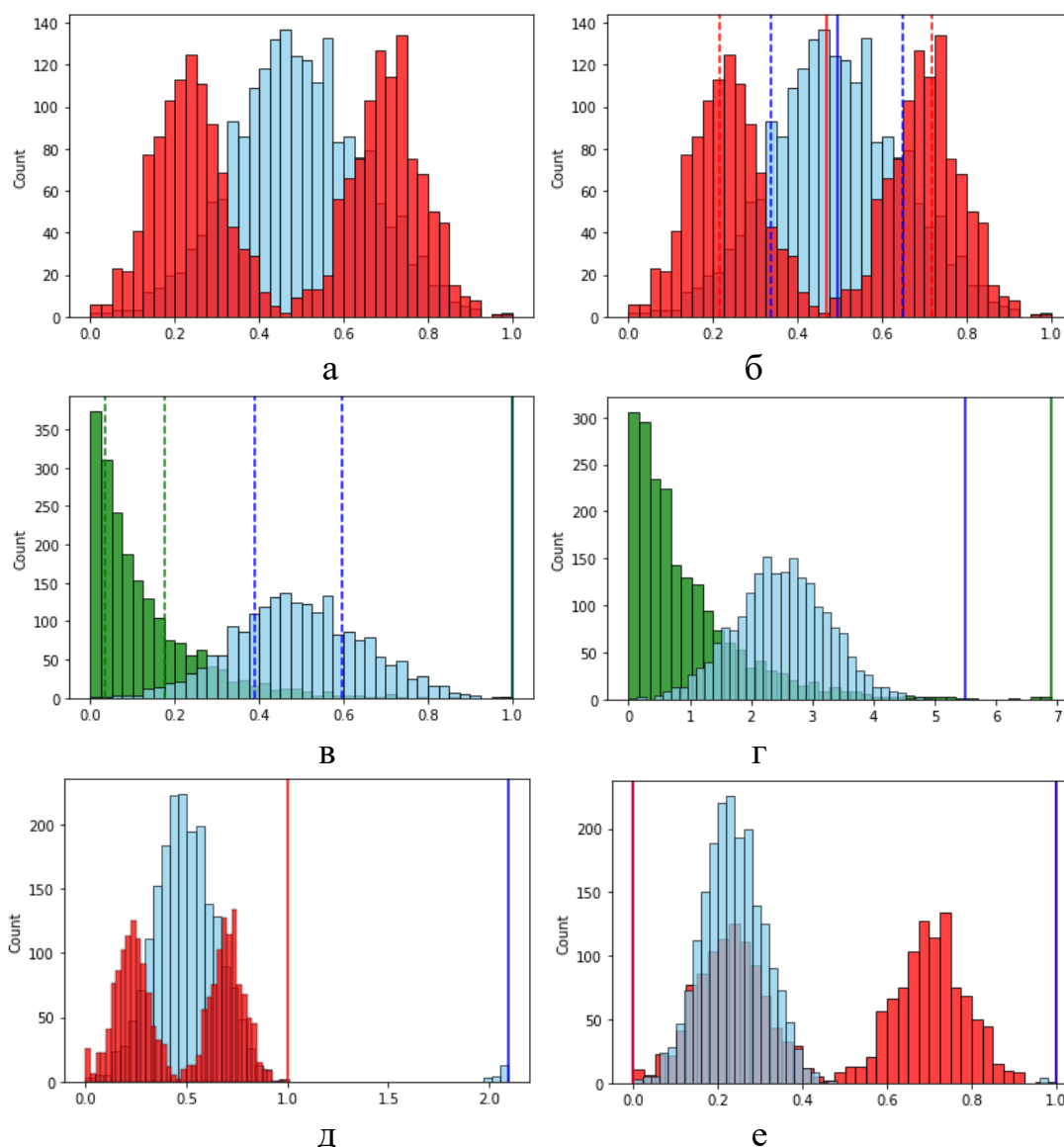
Рис. 5.3. К выбору интервала для масштабирования: а, в, д – исходные распределения; б, г, е – распределения после масштабирования (источник [ https://habr.com/ru/articles/527334/ ])
