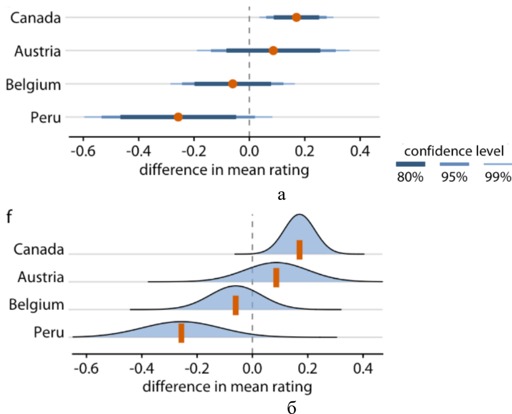
Рис. 4.31. Средние оценки вкуса шоколада для производителей из четырех разных стран относительно средней оценки плиток шоколада из США: а – доверительные интервалы с градуировкой по значениям; б – доверительные распределения [ https://clauswilke.com/dataviz/visualizing-uncertainty.html ]
