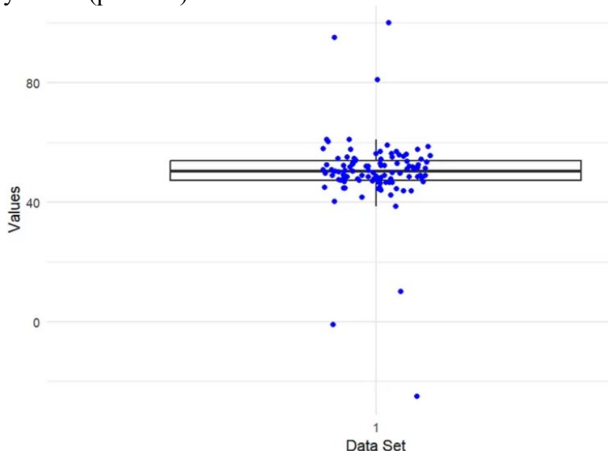
Рис. 4.4. Определение аномалий по методу Тьюки (источник [ https://medium.com/data-and-beyond/outlier-detection-in-r-tukey-method-or-why-you-need-box-and-whiskers-3c35d9ad8fb3 ])
