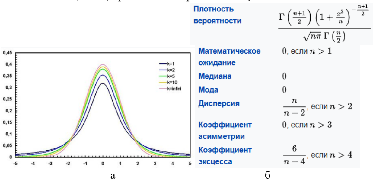
Рис. 3.21. Распределение Стьюдента: ФПР (а) и числовые характеристики (б);
