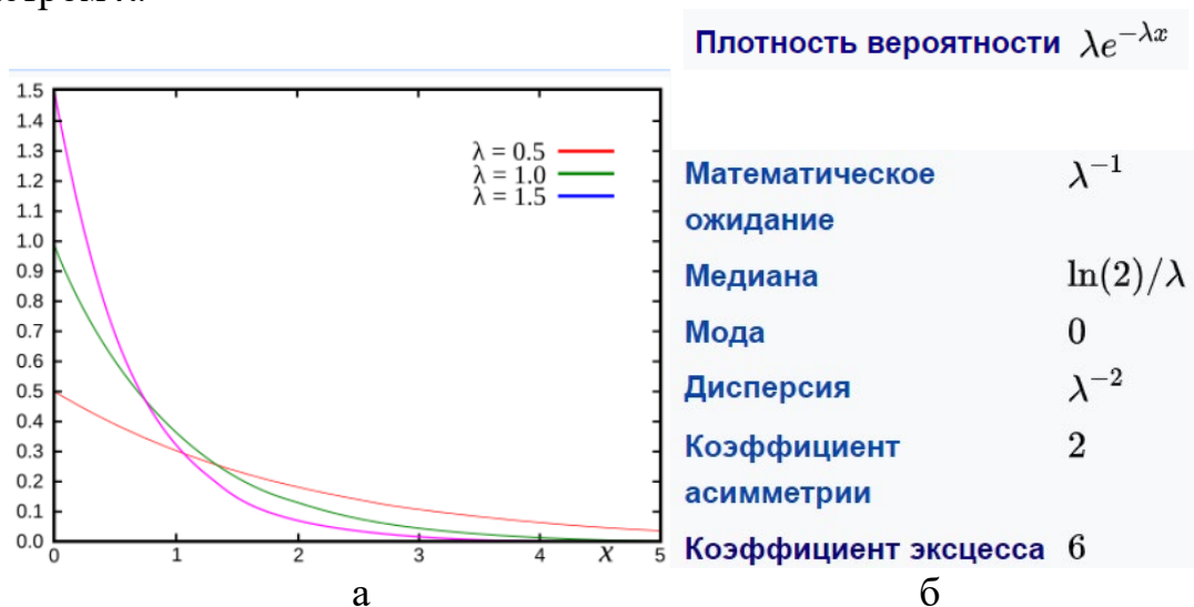
Рис. 3.17. Экспоненциальное распределение: ФПР (а) и числовые характеристики (б) (источник [https://ru.wikipedia.org/wiki/Экспоненциальное_распределение])
