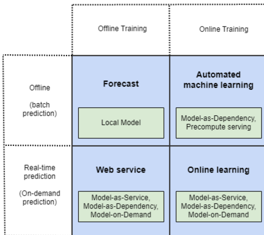
Рис. 7.3. Варианты развертывания модели (источник [https://habr.com/ru/articles/795985/])
