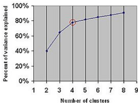
Рис. 6.6. Метод локтя для расчета числа кластеров (источник [ https://neptune.ai/blog/ml-model-evaluation-and-selection ])
