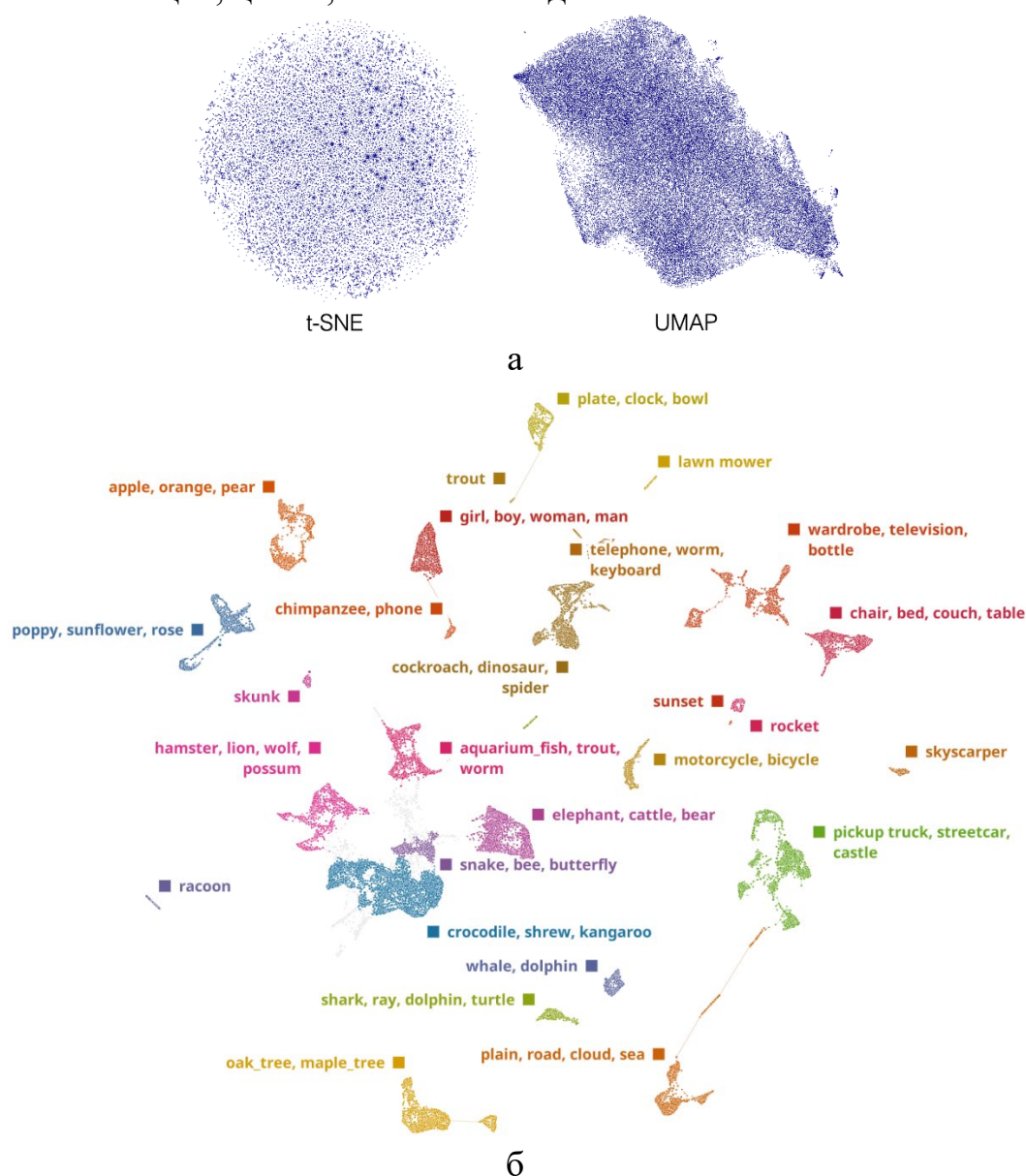
Рис. 2.8. Кластеризация изображений: а – традиционные алгоритмы, б – DTA
