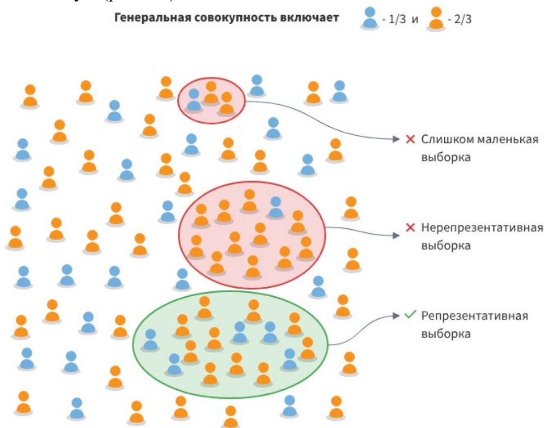
Рис. 3.1. Качественная и количественная репрезентативность выборки
