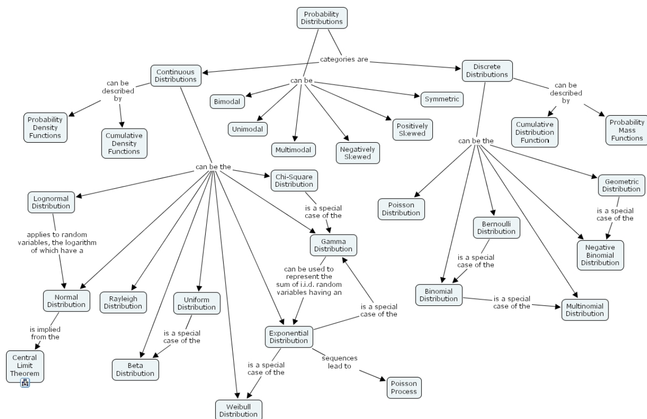
Рис. 3.9. Функции распределения вероятностей и их взаимосвязь (источник [https://skat.ihmc.us/rid=1110240761600_1633886338_5337/Probability_Distributions.cmap])
