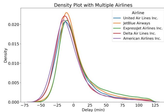
Рис. 4.39. Вид плотности распределения переменной по нескольким категориям
