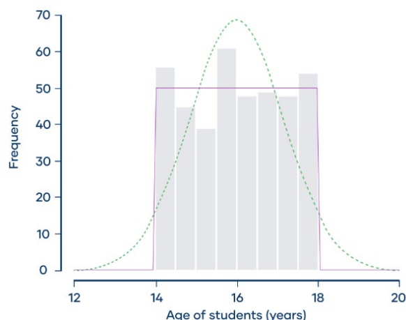
Рис. 3.11. К выбору плотности вероятности по гистограмме (источник [https://www.scribbr.com/statistics/kurtosis/#:~:text=Kurtosis%20is%20a%20measure%20of,(thin%20tails)%20are%20platykurtic])
