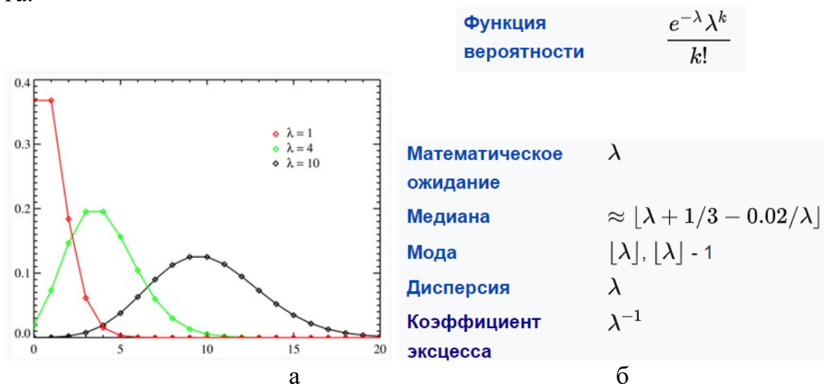
Рис. 3.16. Распределение Пуассона: ФПР (а) и числовые характеристики (б) (источник [ https://ru.wikipedia.org/wiki/Распределение_Пуассона ])
