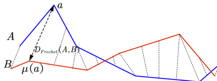
Рис. 3.17. К расчету расстояния Фреше (источник [Guo])
