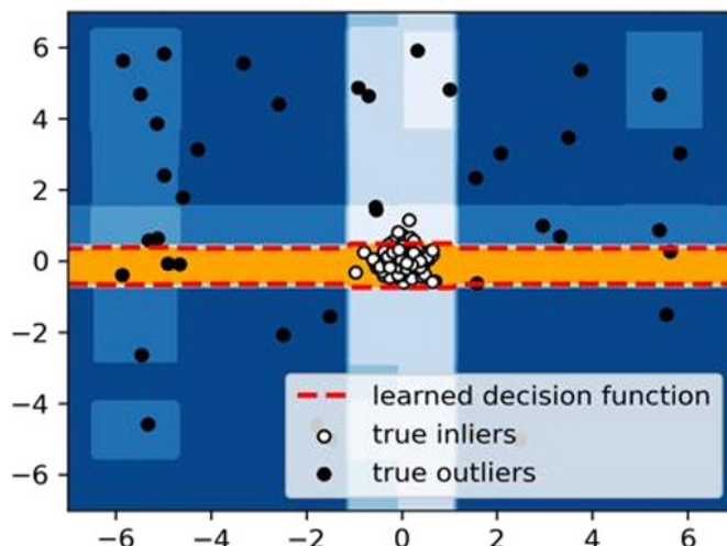
Рис. 4.5. Определение выбросов по гистограммному методу (источник [Sikder])
