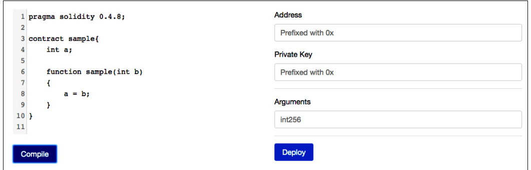
Рис. 6.2. Экран приложения после ввода кода контракта и нажатия кнопки Compile
