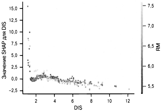
Рис. 16.4. График зависимости для DIS. Если DIS не очень мало, график SHAP остается относительно плоским
