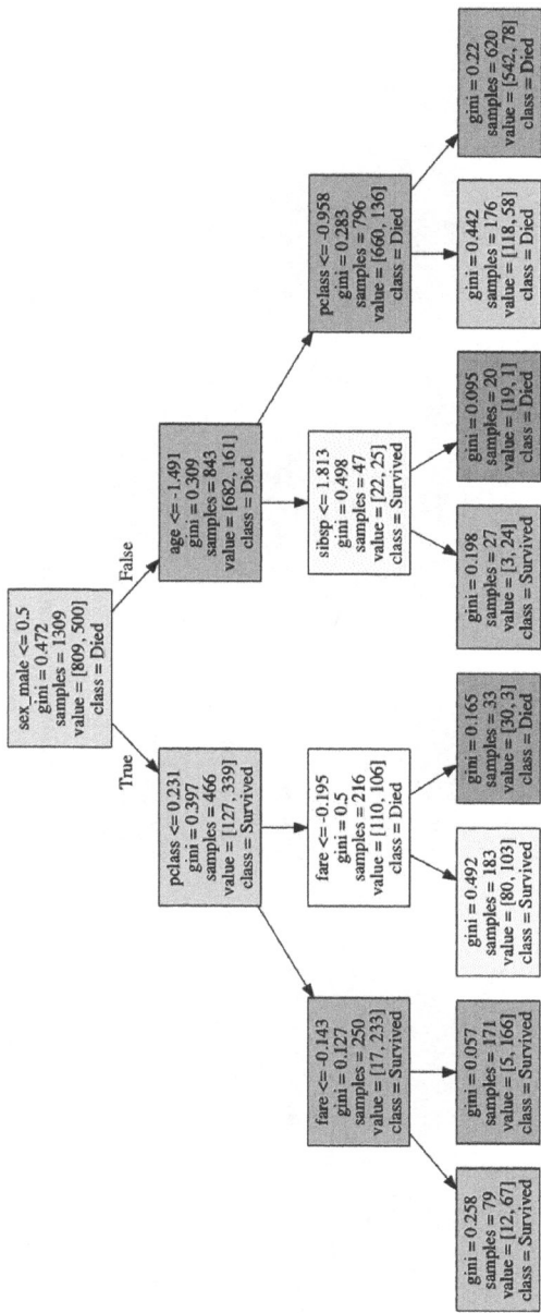
Рис. 10.2. Дерево решений
