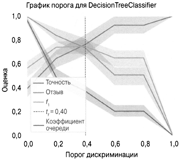
Рис. 12.10. Порог дискриминации
