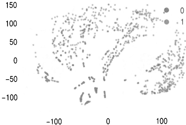
Рис. 17.18. Результаты PHATE
