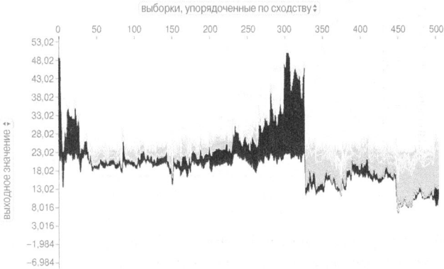
Рис. 16.2. График силы для регрессии по всем выборкам
