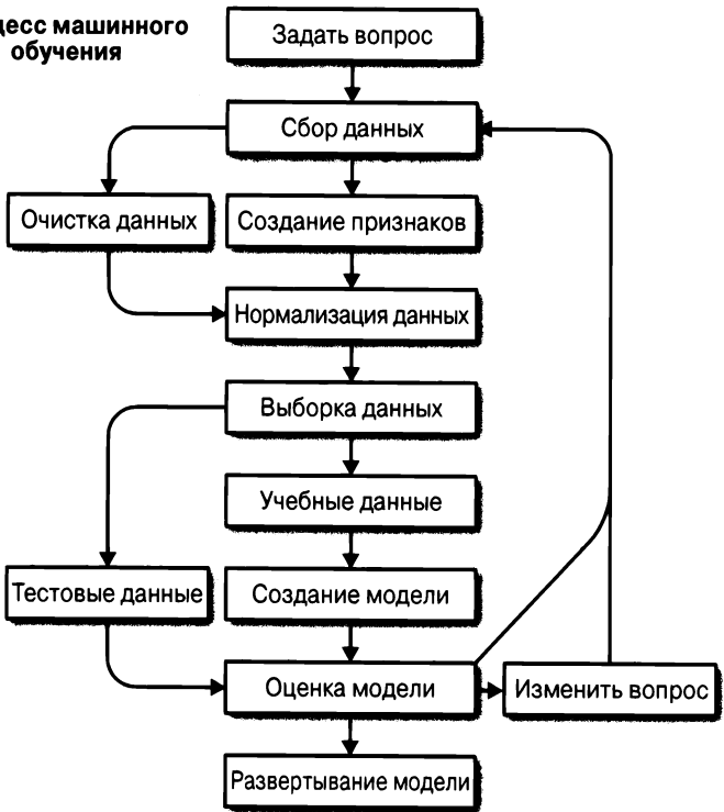
Рис. 2.1. Общий рабочий процесс машинного обучения
