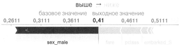
Рис. 13.4. Вклады признаков Shapley для выборки 20. На этом графике показаны базовое значение и признаки, способствующие гибели
