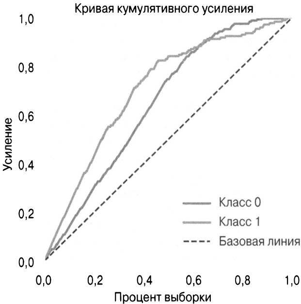
Рис. 12.6. Кривая кумулятивного усиления. Если бы мы упорядочили людей на Титанике в соответствии с нашей моделью, рассмотрим 20% из них, мы получили бы 40% выживших
