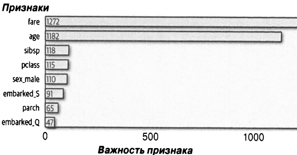
Рис. 10.8. Важность признака, разделенная для LightGBM
