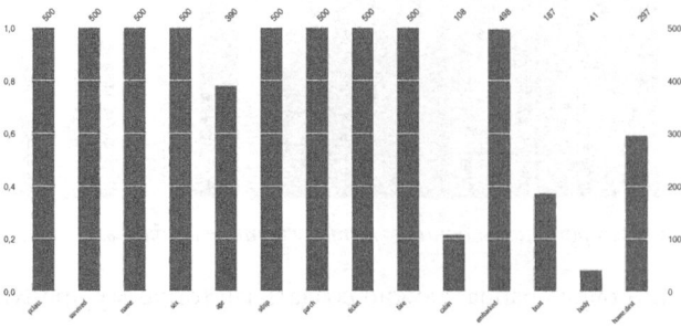
Рис. 4.3. Процент присутствующих и пропущенных данных
