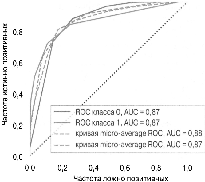
Рис. 12.4. Кривая ROC
