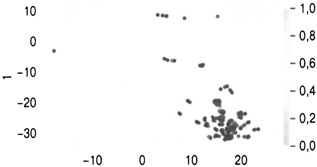
Рис. 17.13. Результаты UMAP
