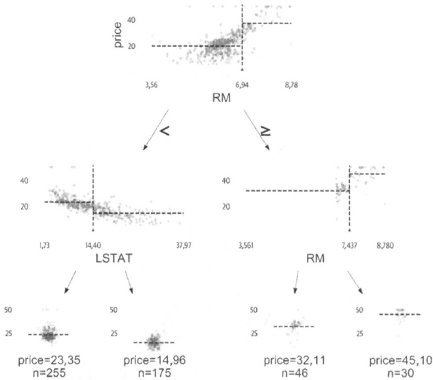
Рис. 14.4. Регрессия dtviz
