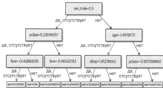
Рис. 10.7. Дерево XGBoost
