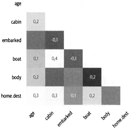
Рис. 4.4. Корреляции присутствующих данных с пропущенными
