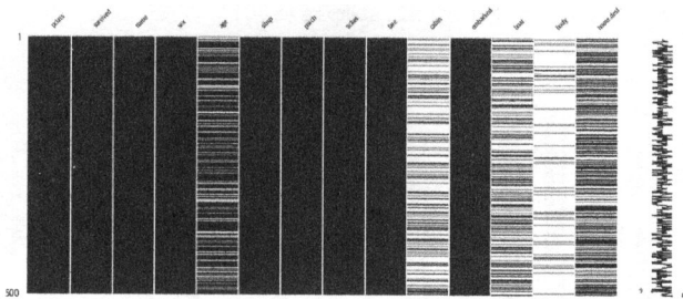
Рис. 4.1. Где пропущены данные. Автору четкие шаблоны не очевидны
