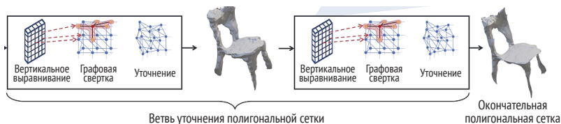
Рис. 10.9 ❖ Ветвь уточнения полигональной сетки
