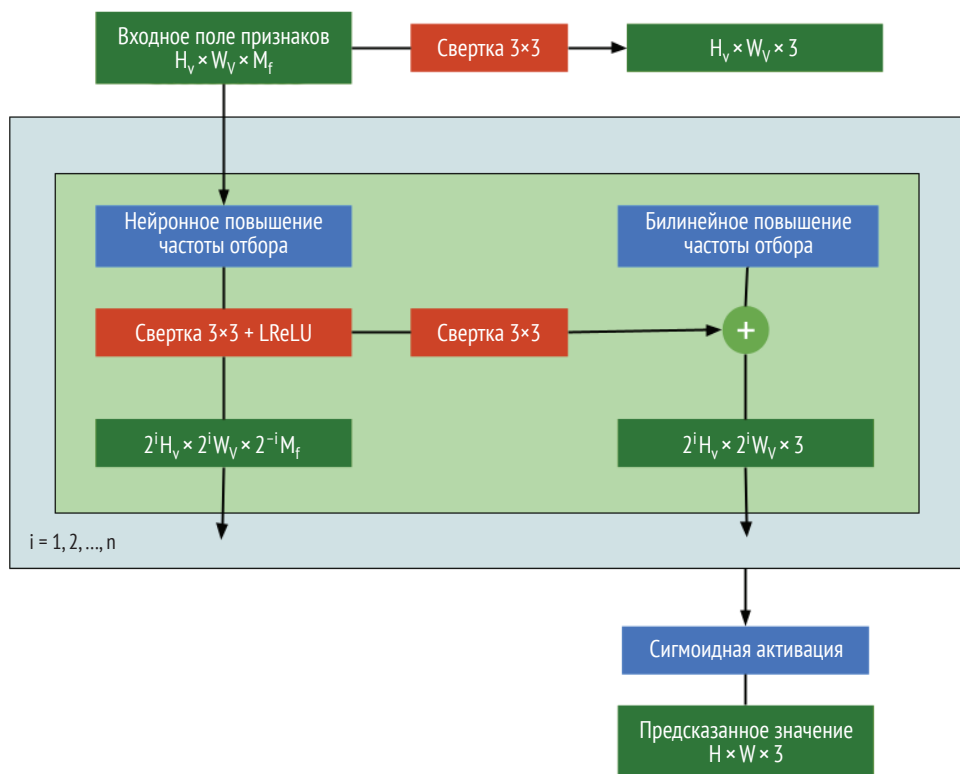
Рис. 7.5 ❖ Модель нейронной отрисовки; это двумерная CNN-сеть с серией операторов повышения частоты отбора ближайших соседей и параллельным отображением в область значений RGB-изображения
