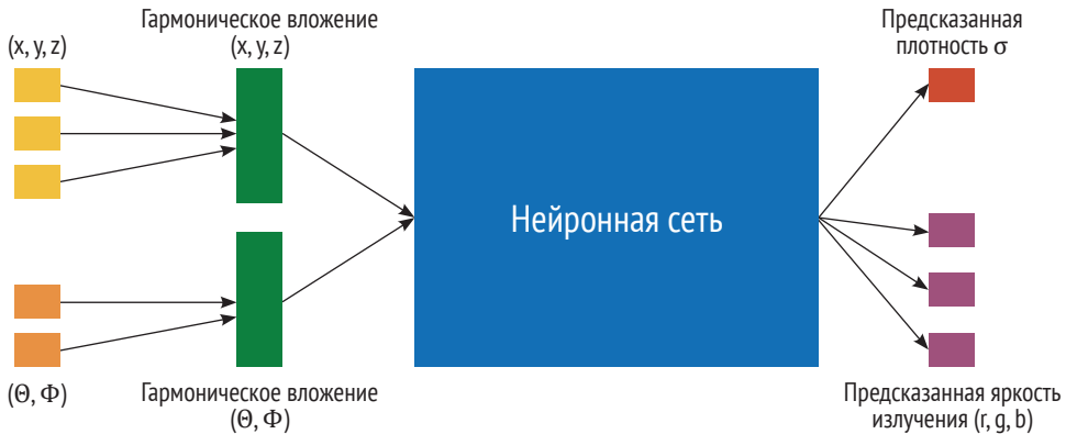
Рис. 6.2 ❖ В начале входные данные (x, y, z, \theta \text{ и } \phi) используются для создания отдельных гармонических вложений для пространственного местоположения и угла обзора, формируя данные, подаваемые на вход в нейронную сеть, и затем эта нейронная сеть выводит предсказанные плотность и яркость излучения
