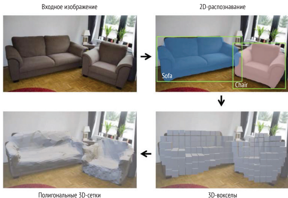
Рис. 10.4 ❖ Общая структура модели Mesh R-CNN
