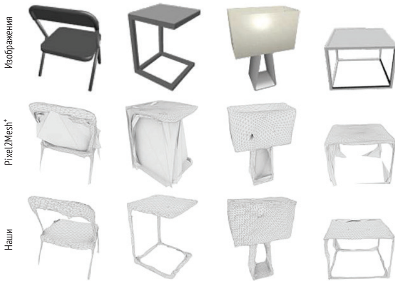
Рис. 10.10 ❖ Предсказатель полигональной сетки на наборе данных ShapeNet
