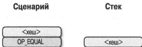
Рис. 13.14. Вторая стадия выполнения сценария p2sh-p2wprkh
