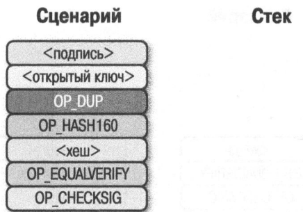
Рис. 6.18. Начальное состояние сценария p2rkh
