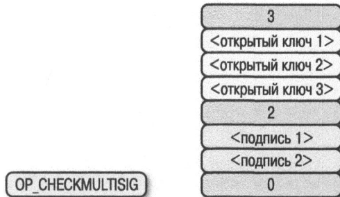
Рис. 13.29. Четвертая стадия выполнения сценария r2wrkh
