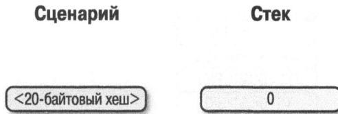
Рис. 13.5. Первая стадия выполнения сценария p2wpkh
