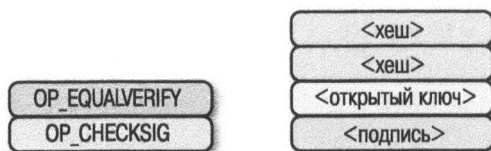
Рис. 6.22. Четвертая стадия выполнения сценария p2rkh
