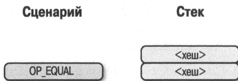
Рис. 13.15. Третья стадия выполнения сценария p2sh-p2wprkh
