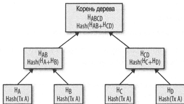
Рис. 11.1. Дерево Меркла
