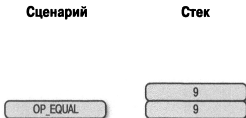
Рис. 6.32. Четвертая стадия выполнения объединенного сценария
