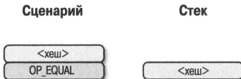
Рис. 13.36. Вторая стадия выполнения сценария p2sh-p2wsh
