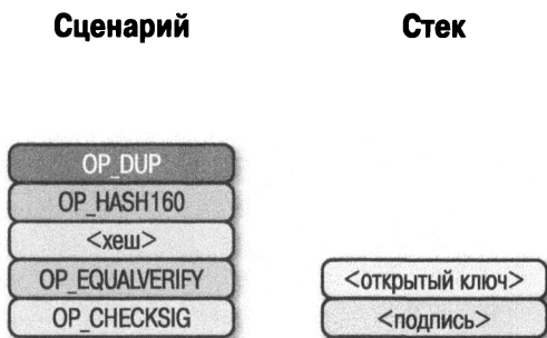
Рис. 6.19. Первая стадия выполнения сценария p2rkh
