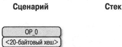
Рис. 13.16. Четвертая стадия выполнения сценария p2sh-p2wprkh
