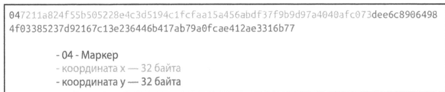
Рис. 4.1. Несжатый формат SEC
