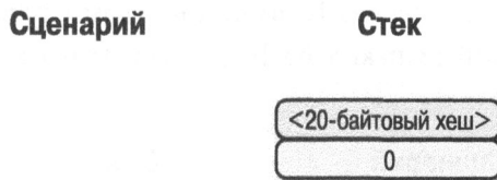
Рис. 13.6. Вторая стадия выполнения сценария p2wpkh
