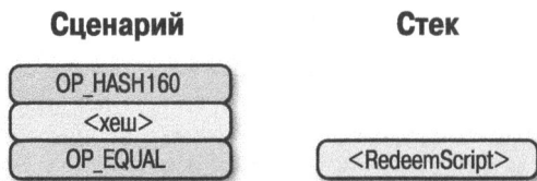
Рис. 13.35. Первая стадия выполнения сценария p2sh-p2wsh
