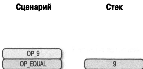
Рис. 6.31. Третья стадия выполнения объединенного сценария
