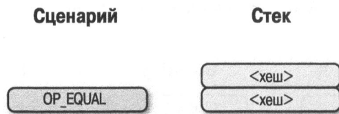
Рис. 13.37. Третья стадия выполнения сценария p2sh-p2wsh
