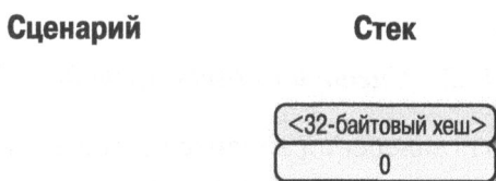
Рис. 13.25. Вторая стадия выполнения сценария p2wpkh
