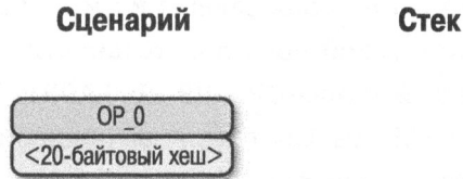
Рис. 13.4. Начальное состояние сценария p2wpkh
